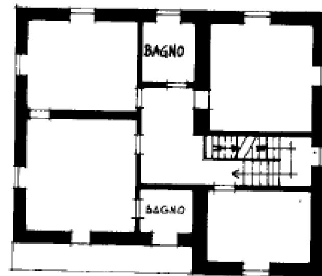
PIANO PRIMO
